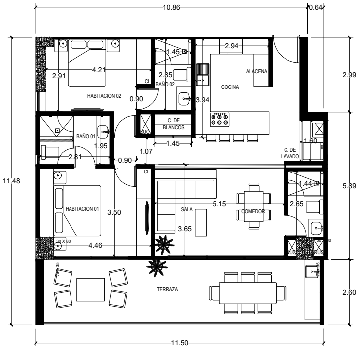
DEPARTAMENTO TIPO CHEL 3
