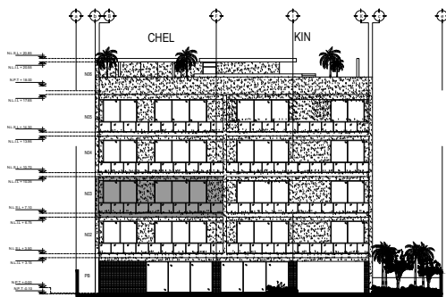
ALZADO POSTERIOR - VISTA JARDIN - TORRE PUEBLO
