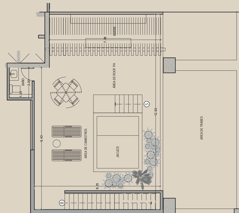
Planta Tipo: Roof Top PH B
